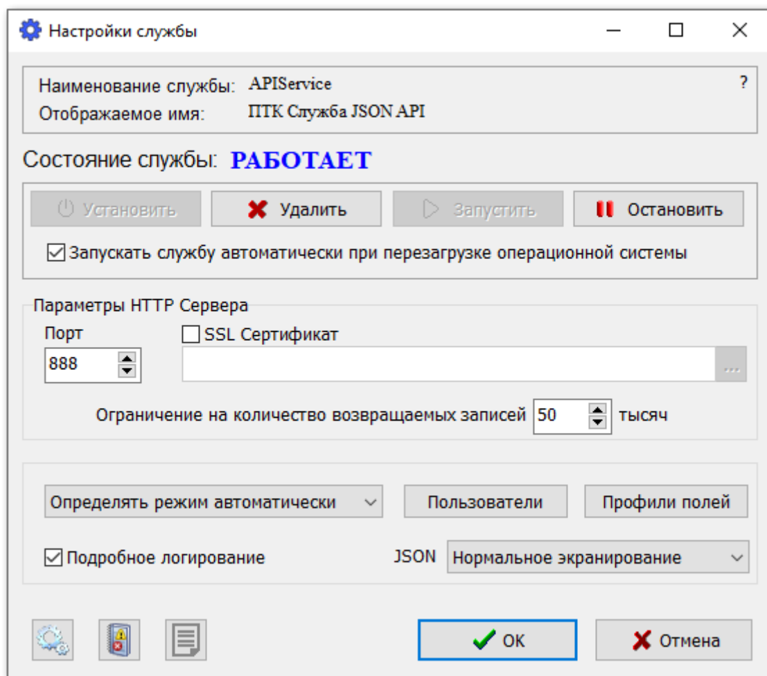
Рис. 7: Служба запущена.
